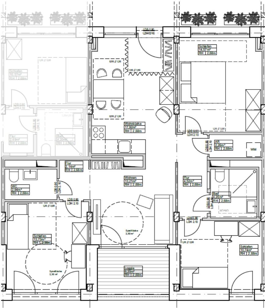
Grundrissdarstellung unter Vorbehalt © kadawittfeldarchitektur
