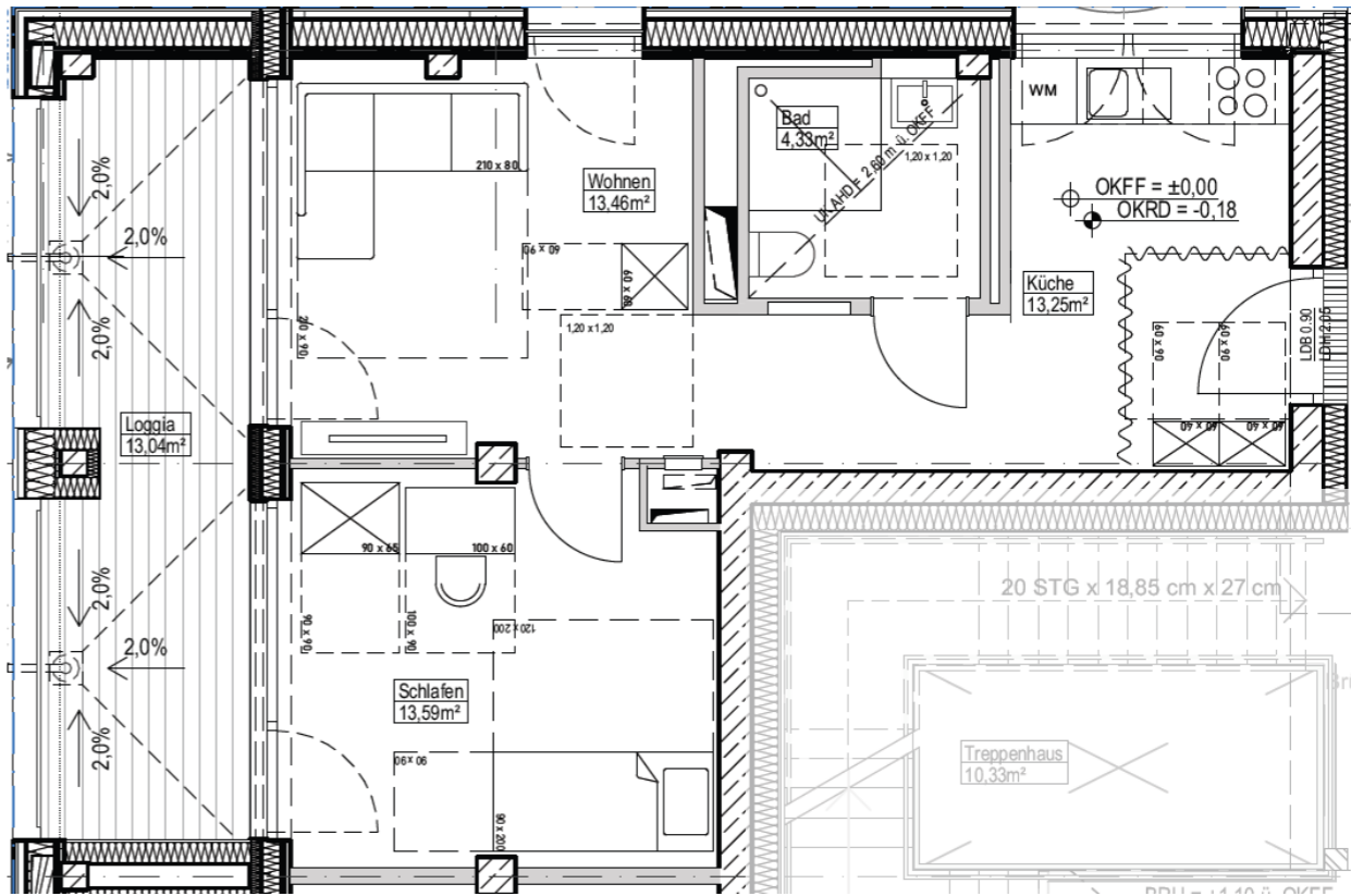
Grundrissdarstellung unter Vorbehalt
