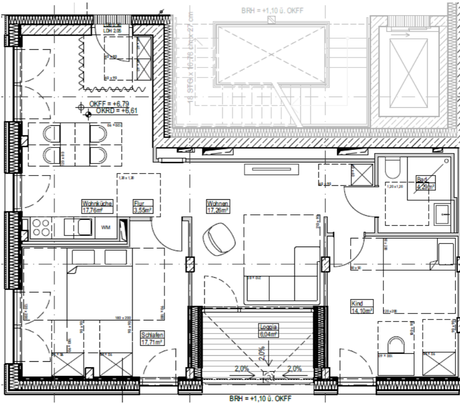
Grundrissdarstellung unter Vorbehalt © kadawittfeldarchitektur
